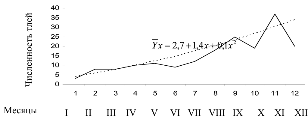
Рис. 2. Линия аппроксимации сезонного изменения динамики численности Tuberolachnus salignus ( P = 0,05 ; t_f = 14,92 ; t_{st} = 16,92 )
